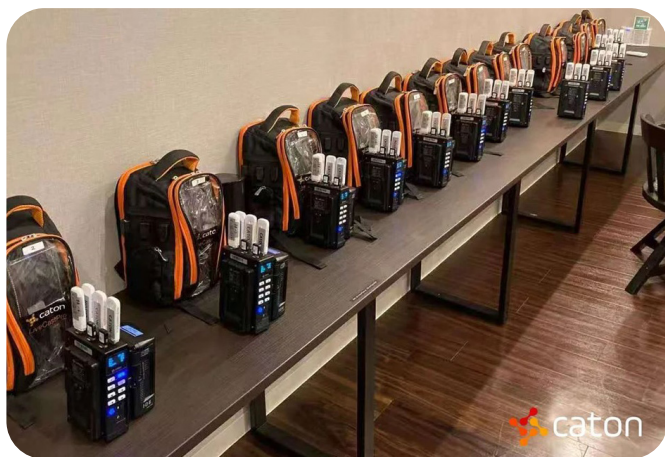
照片：科腾移动编码器已准备好部署到现场记者
