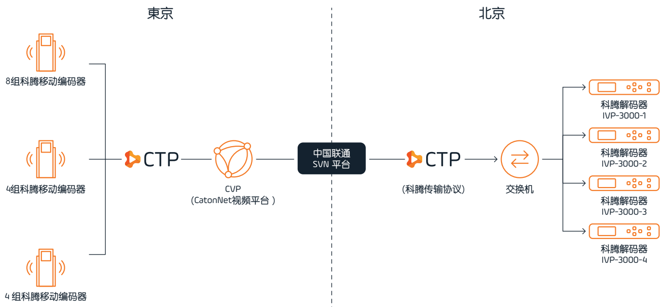
Caton科腾2020东京奥运会实时视频传输方案
